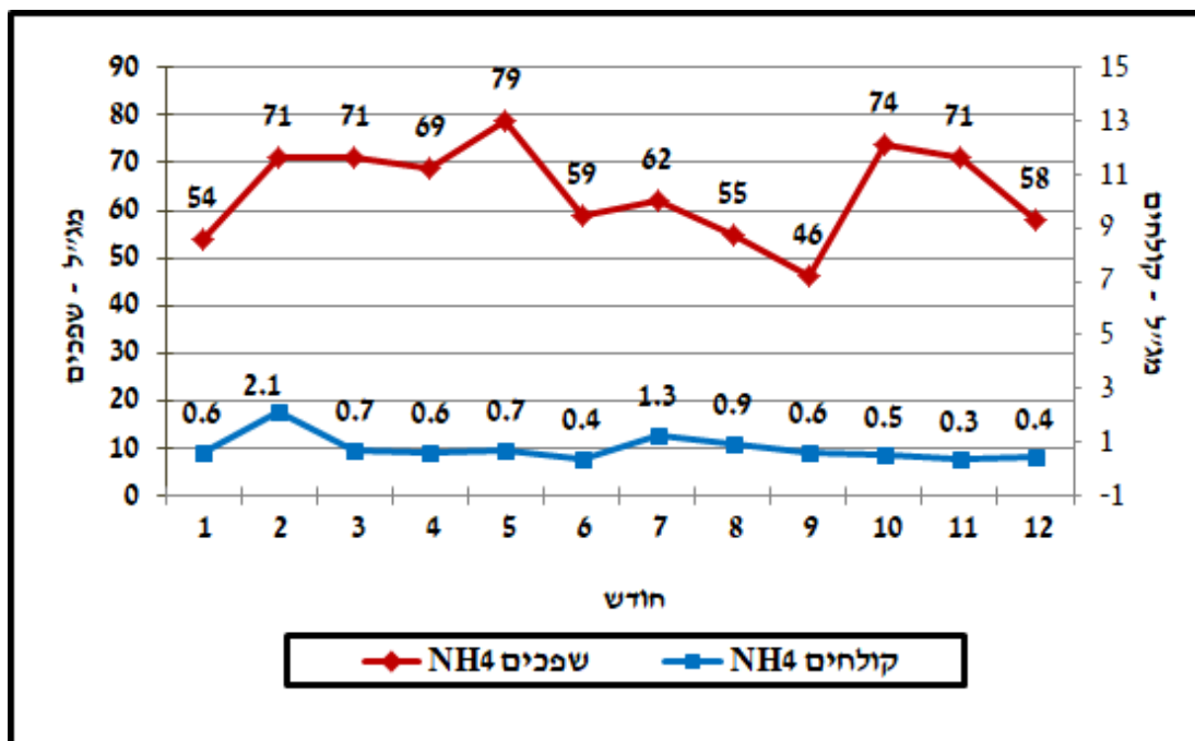
איור מס' 13: ריכוז חנקן אמוניקלי ( N-NH_4 ) בשפכים ובקולחים 2018
