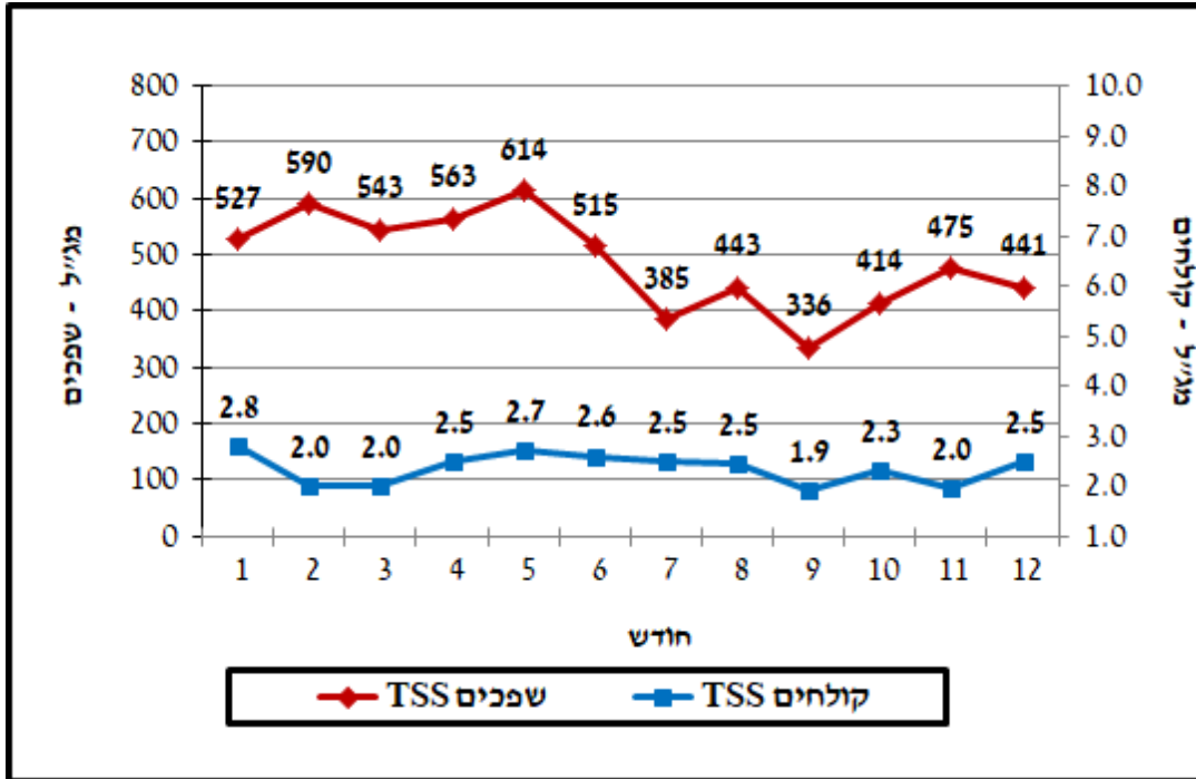
איור מס' 11: ריכוז מוצקים מרחפים ( TSS_{105} ) בשפכים ובקולחים 2018
