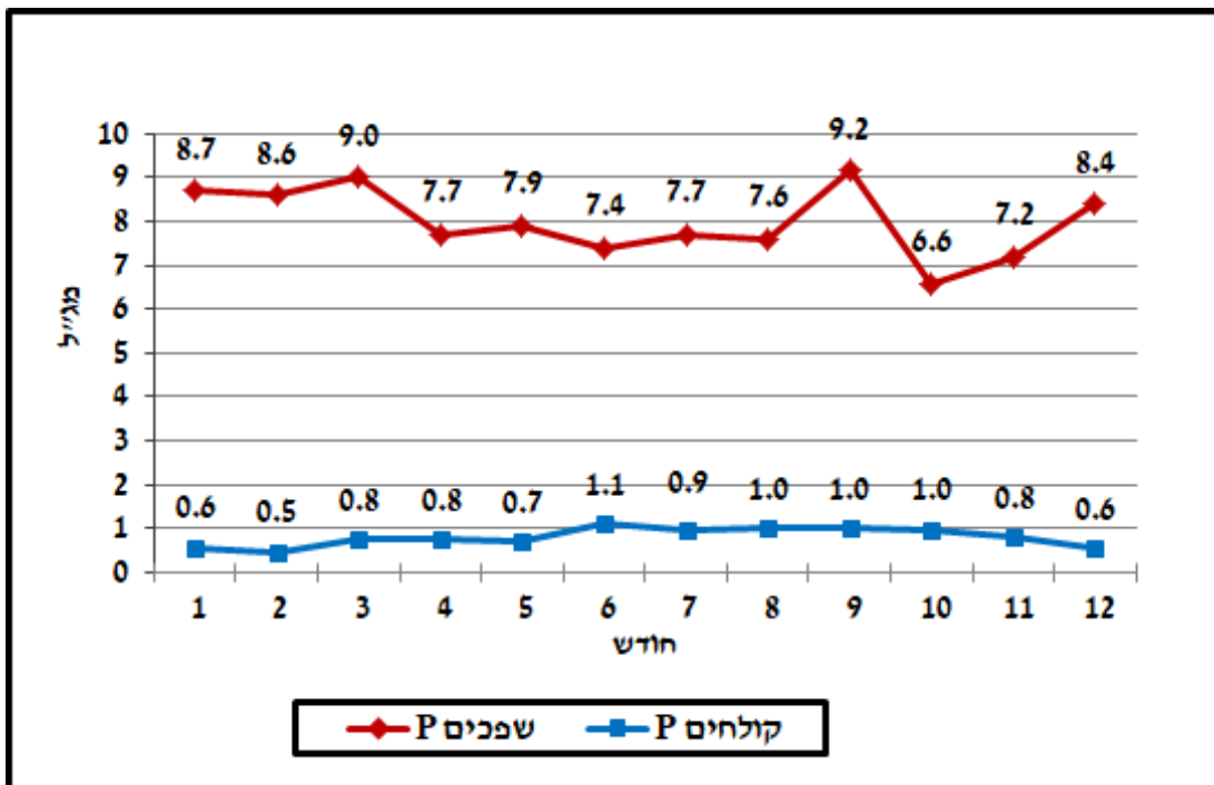
איור מס' 12: ריכוזי זרחן ( P_T ) בשפכים הגולמיים ובקולחים 2018
